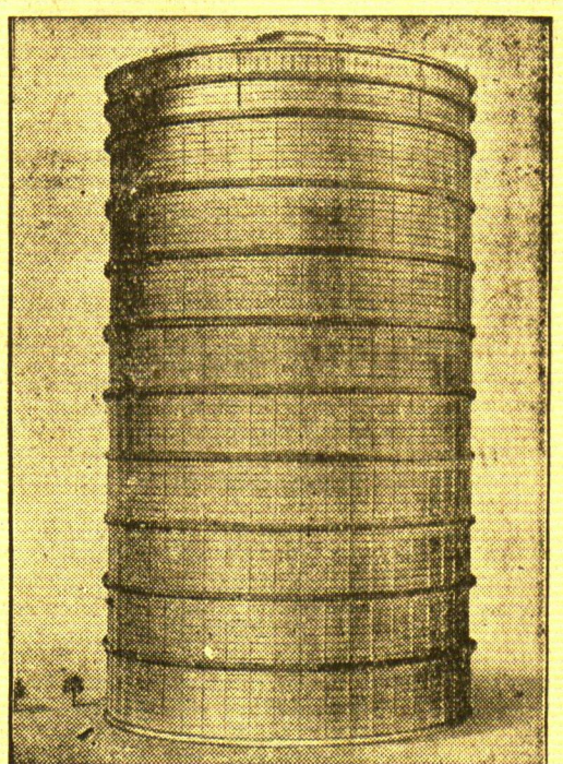
Der größte Gasbehälter der Welt erhebt in Gelsenkirchen
