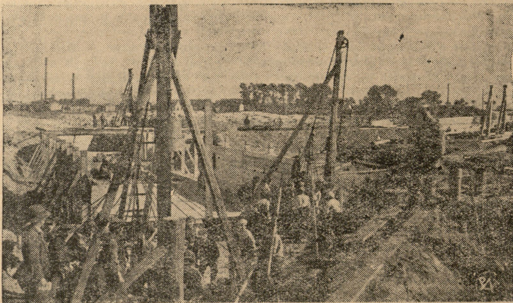
Zdjęcie nasze przedstawia fragment wielkich robót, zorganizowanych przez Fundusz Pracy przy regulacji rzeki Czarnej Przemszy pod Sosnowcem. Na robotach tych, prowadzonych na odcinku 16 klm. jest stale zatrudnionych około 1000 robotników.
