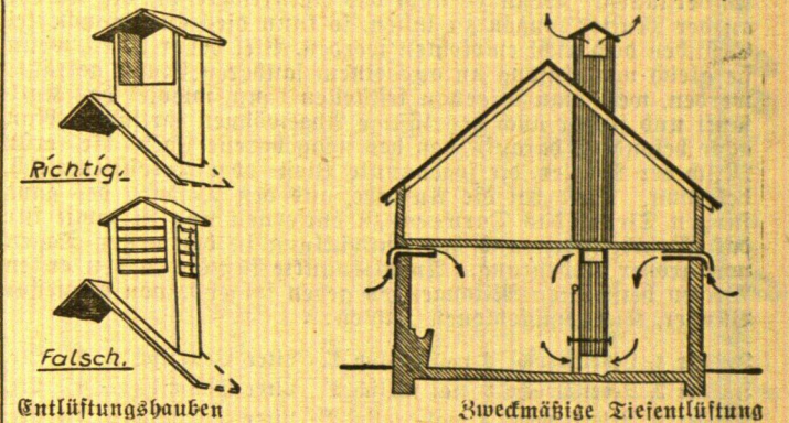
Entlüftungshauben Zweckmäßige Tiefentlüftung
