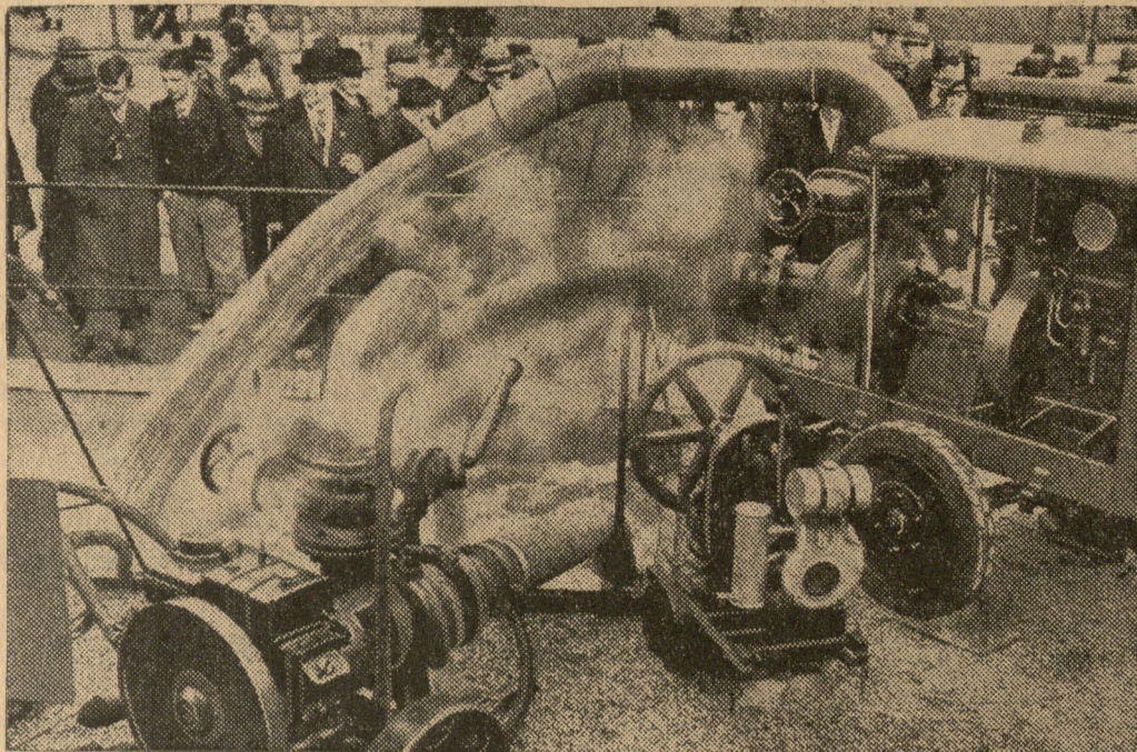
Pompa irygacyjna, wystawiona na targach lipskich, która w znacznym stopniu uniezależnia od warunków atmosferycznych, pozwalając w krótkim czasie orosić znaczne obszary.
