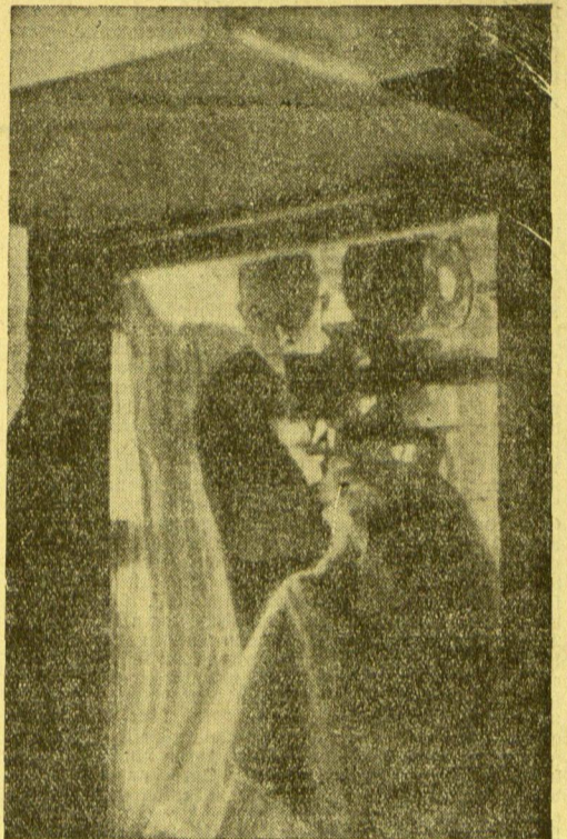
Die Tonfilmkamera ist in einem durch Glas abge-schlossenen Kasten eingebaut, um sie vor ungewünschten Geräusch-Einflüssen zu schützen.
