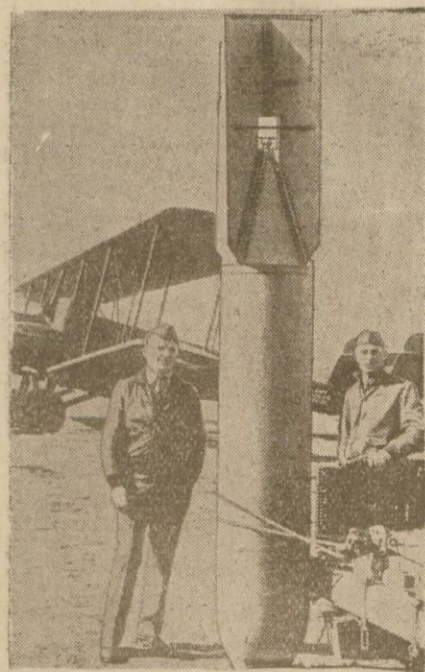
Bomba lotnicza t. zw. „Gruba Berta“ wysokości 3 mtr.
