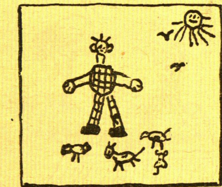
Ein Bildchen für die Tiernummer von unserer jüngsten Mitarbeiterin
