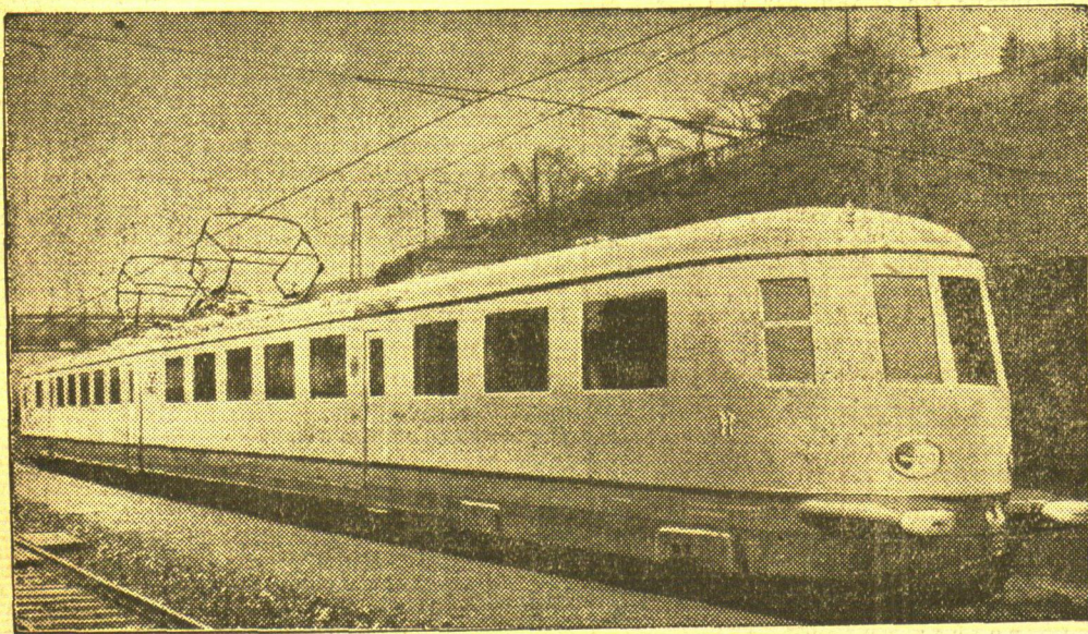
Links: In 5 Stunden von Berlin nach München. Der neue elektrische Schnelltriebwagen der Deutschen Reichsbahn. Die Deutsche Reichsbahn bildet jetzt eine elektrische Lokomotive durch, die auf der Strecke Berlin-München eingesetzt werden soll, sobald die Elektrifizierungsarbeiten beendet sein werden. Mit dieser Maschine sollen dann die FDs-Züge mit einem Stundendurchschnitt von 180 Kilometer fahren. — Mitte: 300 Jahre Universität Utrecht. In Utrecht fanden aus Anlaß des 300-jährigen Bestehens der Universität große Feiern in der Domkirche statt, an denen auch die Königin der Niederlande teilnahm. Bei ihrem Eintreffen wurde die Königin, wie auf unserem Bild zu sehen ist, von dem Rektor der Universität begrüßt. Eine Ehrenkompanie erwies die Ehrenbezeugung. — Rechts: Farmer demonstrieren in London. 3000 englische Bauern aus allen Landesteilen protestierten am Mittwoch in einem großen Demonstrationsszuge gegen die Kirchensteuern. Eine Geleesvorlage steht die Umlegung des Kirchenscheitens auf die Landwirtschaft vor. — Ein Teilnehmer an der Demonstration, der seine Kopfbedeckung mit Lehren geschmückt und einem Protestplakat versehen hat.
