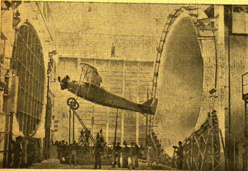
Links: Der größte Windkanal der Welt
