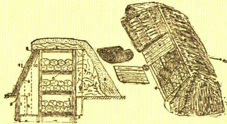
Abb. 1: Einfache, etwa 50 Ztm. in die Erde gesetzte Kohlhütte mit drei Lagerstufen
