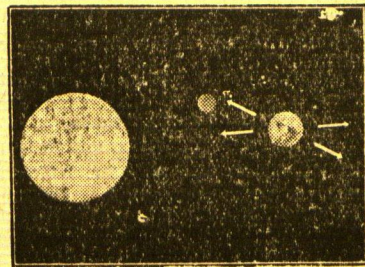
Sonne — Mond — Erde
