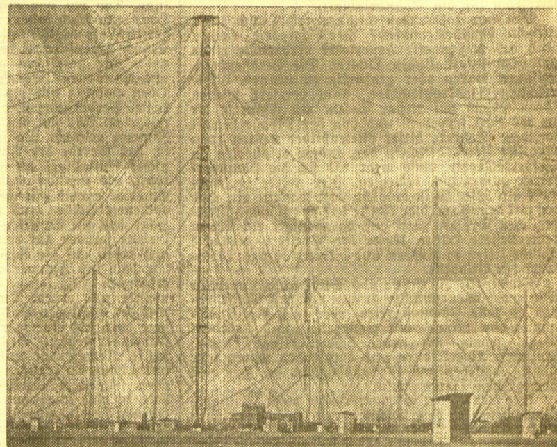
Weit ins Land ragen die Masten der Großfunkstelle Nauen
