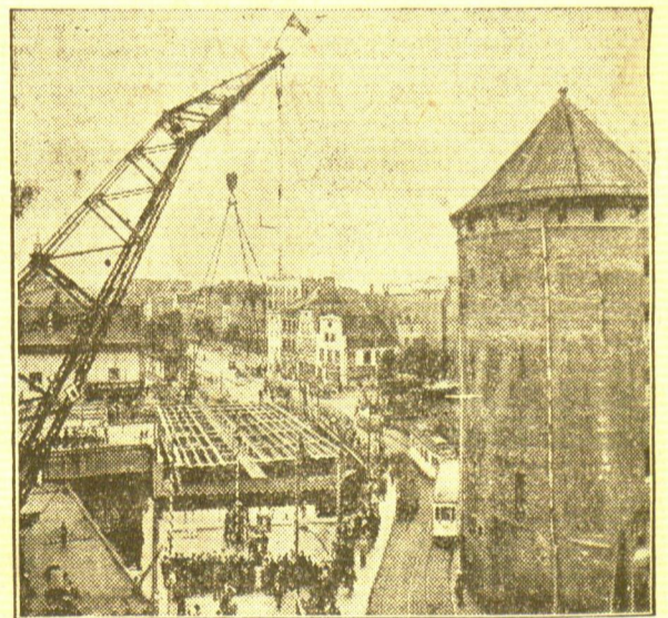
Brückenbau über die Motflan in Danzig
