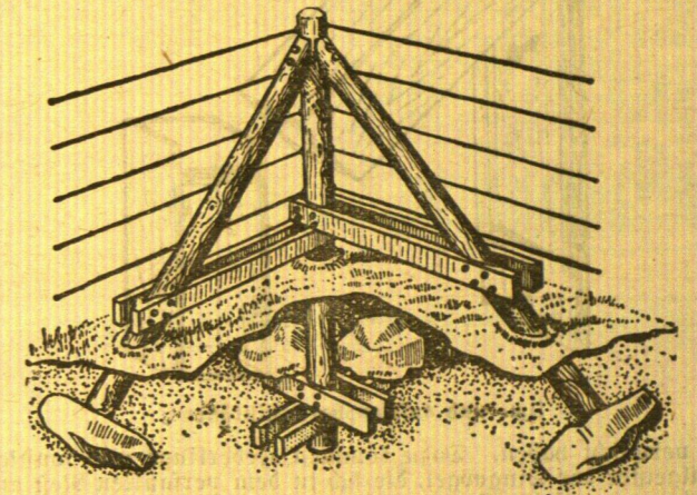
Versteifung eines Stäbelpfostens
