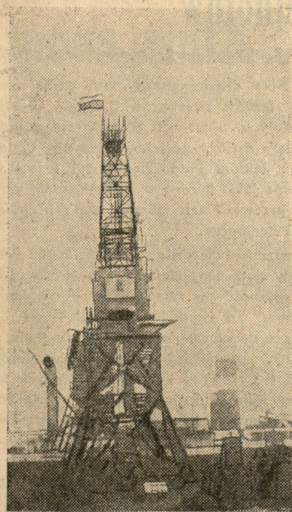
Stale rozrastający się port gdyński otrzymał ostatnio nowy najzupełniej nowoczesny urządzone dźwig o nośności 7 ton, przy szybkości załadunku 140 ton na godz. Dźwig, którego fotografię reprodukuje, został zbudowany przez firmę „Progres”.
