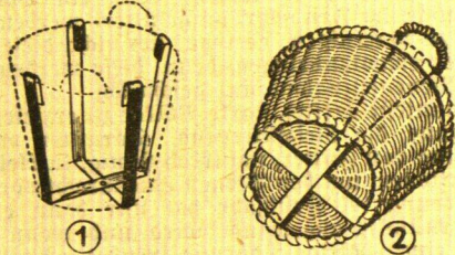
Bandeisen (Abb. 1) und Holzleisten (Abb. 2) verstärken das Geflecht der Weidenkörbe.
