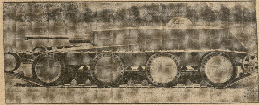
Najnowszy tank amerykański. Model tanka, który może być przymontowany do samolotu i przenoszony w ten sposób drogą powietrzną.
