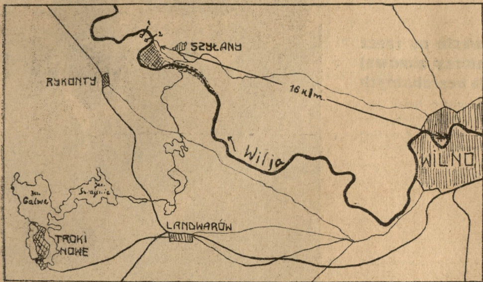
1 — miejsce budowy zapory, według projektu zarządu miejskiego; 2 — miejsce bud. zapory zaproponowane przez prof. Pomianowskiego i nac. Herbichta. Obok i wzdłuż rzeki — zakreślane — miejsce zalewu
