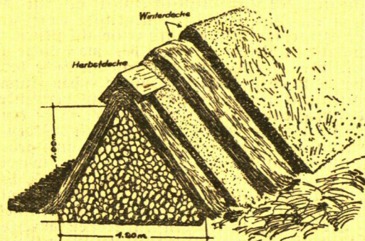
Querschnitt durch eine Kartoffelmiete
