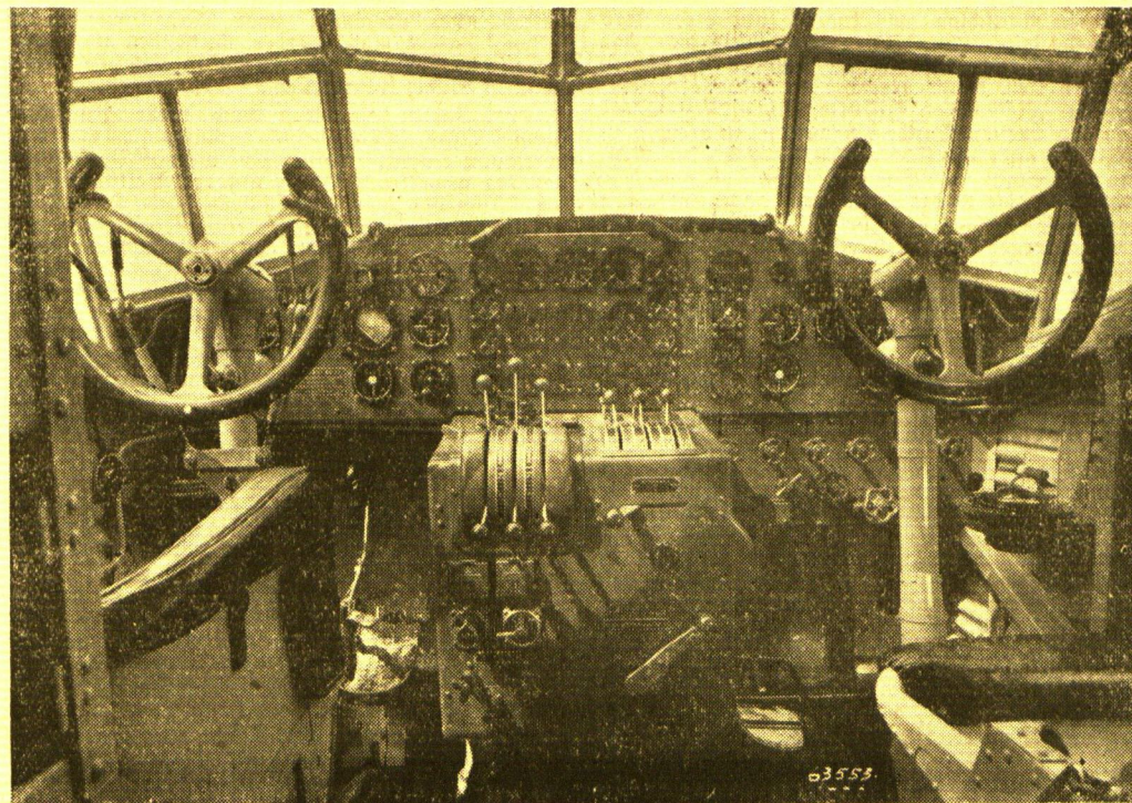
So sieht der Führerstand eines dreimotorigen Verkehrsflugzeuges, der Junkers Ju 52/3 m, aus. Unser Bild zeigt eine Reihe von Geräten für den Blindflug, wie: Fernkompaß, Kurskreisel, Horizontgerät, Wendezähler, Drehzahlmesser usw. (Deutsche Luft Hansa A. G.)
