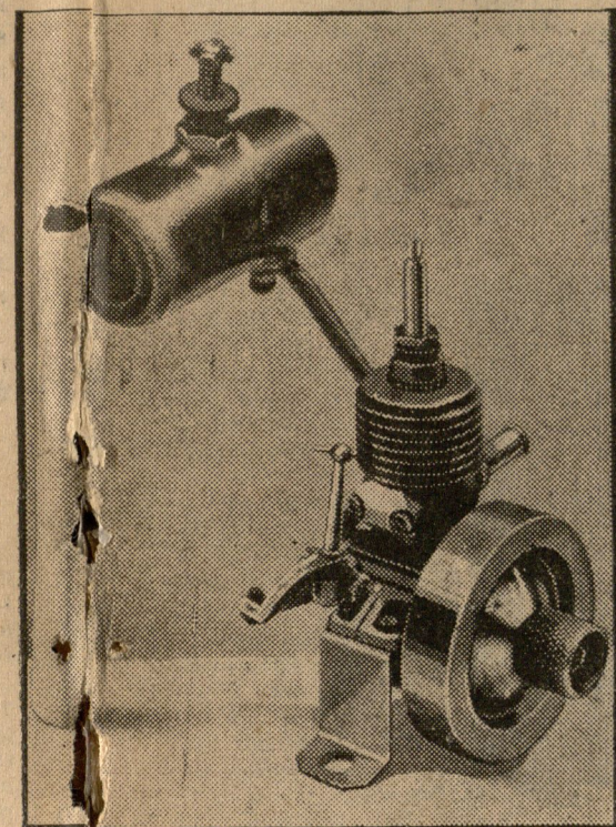
Najmniejszy motor na świecie, został wystawiony na wywiesie wynalazków w New-Yorku. Wysokość tego motoru równa się wysokości papierosa. Zbudowany on jest jednak tak praktycznie, że jego kołowa prędkość daje 5000 obrotów na minutę.
