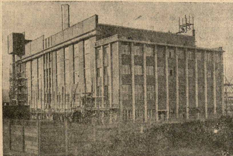
Zdjęcie nasze przedstawia widok ogólny nowej elektrowni w Gdyni, poświęconej w dniu wczorajszym. Elektrownia ta, wyzyskana obecnie w 40%, dostarczyć może energii elektrycznej o mocy 7,500 kilowatów.
