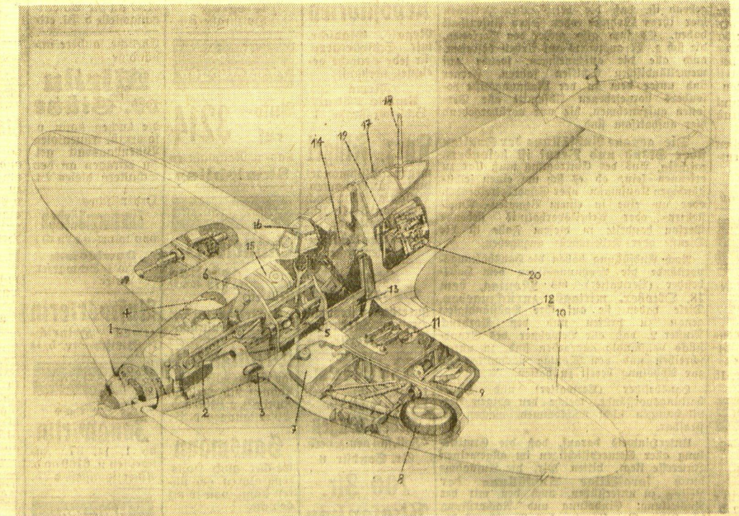
Perspektivische Uebersicht des Jagdeinsitzers Heinkel „He 112“ 1. Motor Jumo 210 Ea; 2. Motorträger; 3. Auspuff; 4. Anlaufschacht für Kompressor; 5. Je 1 MG. auf jeder Seite der Rumpfspitze; 6. Brandschott; 7. Flügelant; 8. Eingeeogenes Fahrwerk; 9. Je 1 Kanone in jeder Flügelhälfte; 10. Querruder; 11. Je 8 Stück 10-kg-Splitterbomben unter jeder
