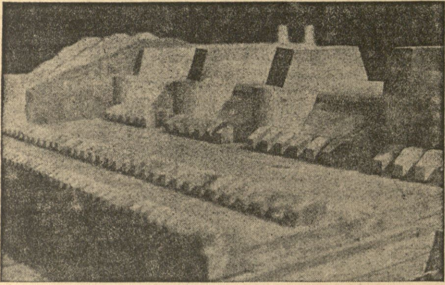
Fragment modelu zapory wodnej w Turniszkach pod Wilnem. Widoczne są trzy stacje przelewowe (żelbetowe) oraz trzy rzędy rozbiijaczy prądu.
