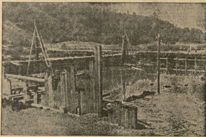
Fragment terenu robót w Turniszkach. Na pierwszym planie budowa jednej ze stacji przelewowych.
