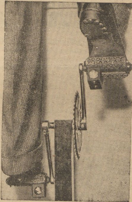
Celem zabezpieczenia kolarzy w nocy przed wzajemnym najeżdżaniem, wprowadzono pedały, które w równomiernych krótkich odstępach, to jest przy naciskaniu świecą i gasną, przez co zwracają uwagę jadącego z tyłu w większym stopniu niż gdyby świeciły stale.
