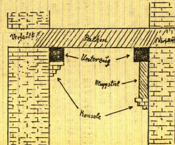
Abstützen schadhafter Dedenbalken
