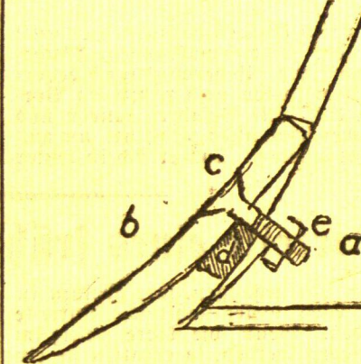
a) Pflugkörper, b) Schar, c) Scharschraube, d) untergelegtes Holz, e) Mutter.
