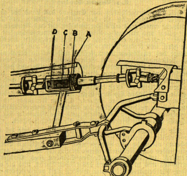
Abb. 3. Rutschkupplung des Zapfwellenantriebes.
