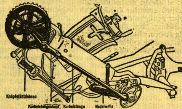
Abb. 2. Kurbelstangenantrieb der Knüpfelnadelwelle.
