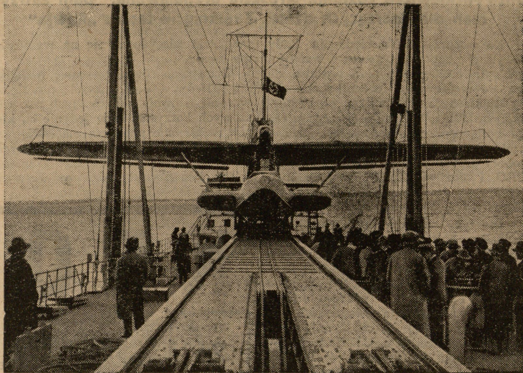
W Kilonji odbyły się próby z trzecią awjomatką niemiecką „Ostmark“, wykończoną 15-go kwietnia r. b. Dwie poprzednio zbudowane, noszą nazwy „Westfallen“ i „Schwabenland“. — Na ilustracji — część pokładu nowej awjomatki z wyrzutnią katapultową, na której stoi przygotowany do startu samolot.
