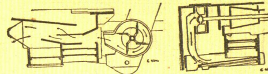
Abb. 1: Pkwert einer Groß-Dreschmaschine (20—35 Ztr. Stb.) mit Druckwind.
