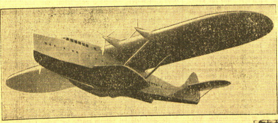
Do 20, ein neues Großflugschiff der Dornier-Werke. Auf Grund der Erfahrungen, die man mit den bisherigen drei Flugschiffen der Do-X-Klasse machte, bauen die Dornier-Werke nunmehr ein neues Flugschiff Do 20, dessen Modell zum erstenmal auf der Internationalen Luftfahrt-Ausstellung in Stockholm der Öffentlichkeit gezeigt wird. Das Flugschiff wird mit acht Dieselmotoren von je 800 bis 1000 PS getrieben und hat bei einer Durchschnittsgeschwindigkeit von 250 bis 300 Kilometerstunden einen Flugbereich von 4000 bis 5000 Kilometer. — Links: Amy Hollison dreifacher Rekord. Die englische Fliegerin Amy Hollison-Johnson lehrte von ihrem Rekordflug nach Kapstadt zurück. Für den Hinflug hatte sie eine neue Bestzeit mit etwas über 3/4 Tagen aufgestellt und ferner auf dem Rückflug sowie in der Gesamtzeit des Hin- und Rückfluges neue Bestleistungen erzielt. Hier sieht man die fröhlich lachende Fliegerin nach ihrer Ankunft mit ihrem Gatten im Wagen.
