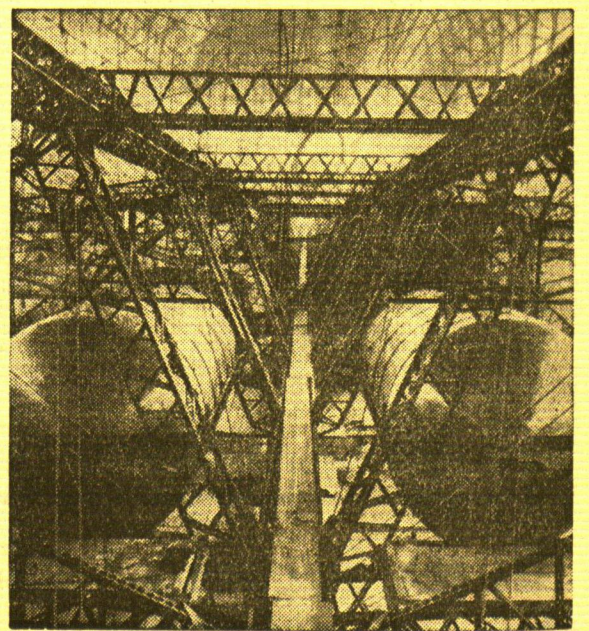
Zeppelin „Z. 3. 129“ im Bau. Neuestes Bild von dem Bau des neuen Zeppelin-Luftschiffes „Z. 3. 129“. Das Bild gewährt einen Blick auf das Gerüst und läßt die ungeheuren Ausmaße dieses Luftschiffes ahnen.
