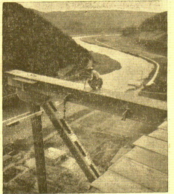
Reichsautobahn-Brückenbau hoch über dem Werratal
