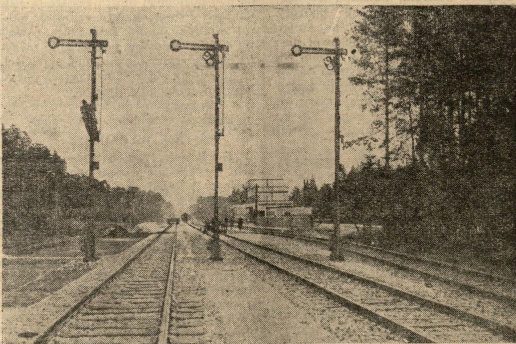
Na Górnym Śląsku odbyła się w obecności min. Komunikacji p. Ulrycha, uroczystość inauguracji nowozbudowanej linii kolejowej Rybnik—Zory, która powstała kosztem 3,300,000 złotych z funduszy skarbu śląskiego. Zdjęcie nasze przedstawia widok ogólny nowej stacji kolejowej Sotartowice, leżącej na nowo otwartej linii Rybnik—Zory.
