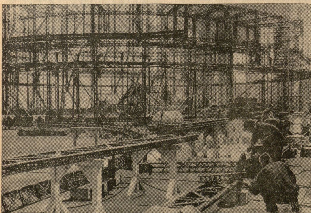
Budowa nowego zeppelinu „LZ 130”.
